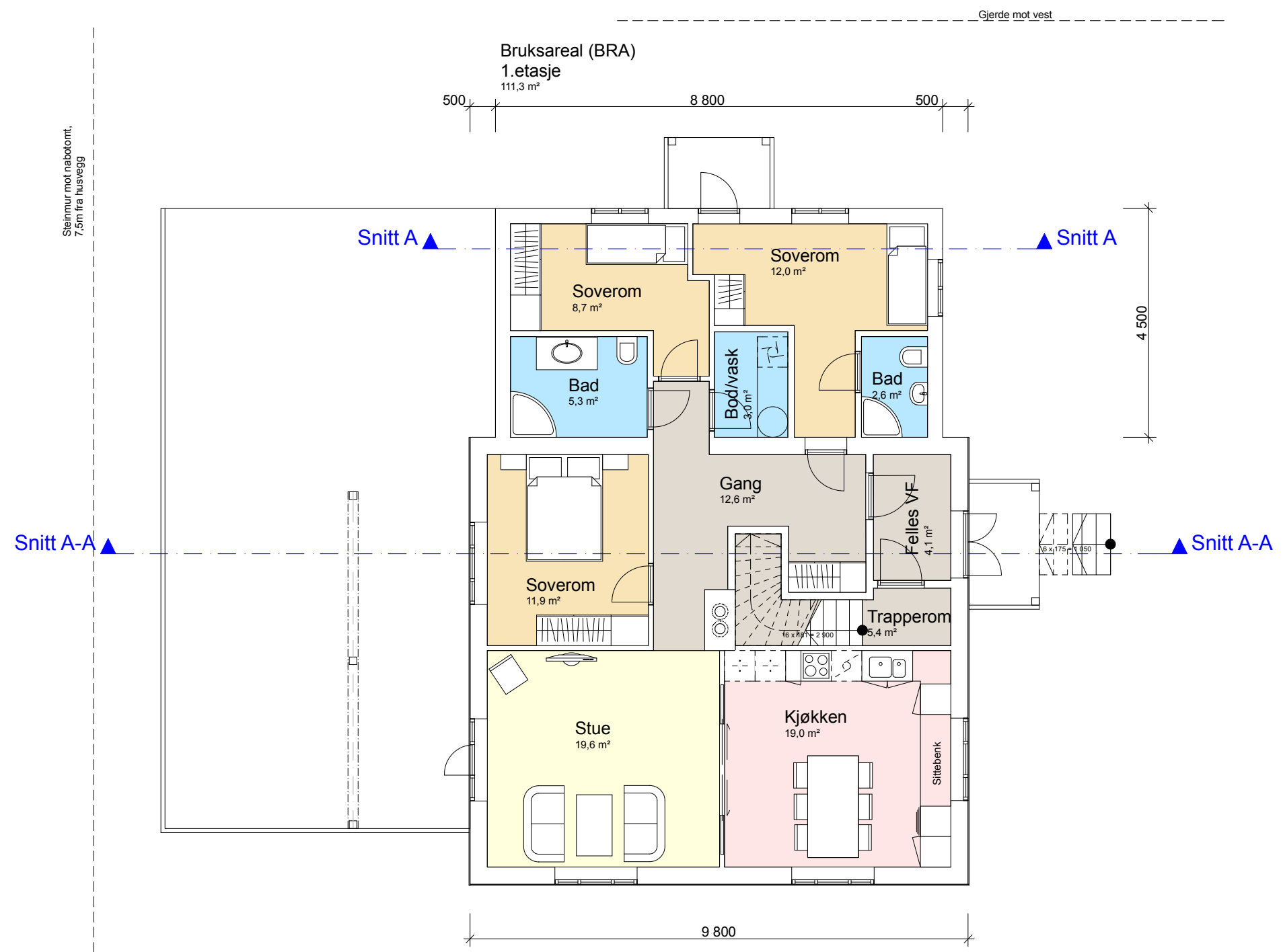
Plan 1.etasje
